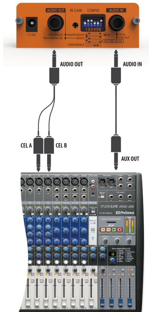
Ilustración 4: Conexión a consola Presonus AR22
