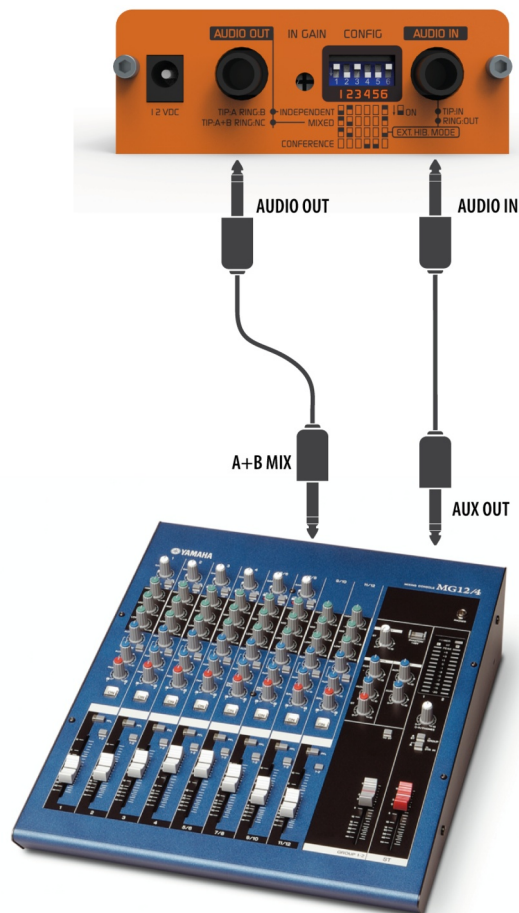
Ilustración 3: Conexión a Yamaha MG12/4
