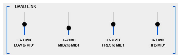
Ilustración 39: MB AGC - Enlace entre bandas
