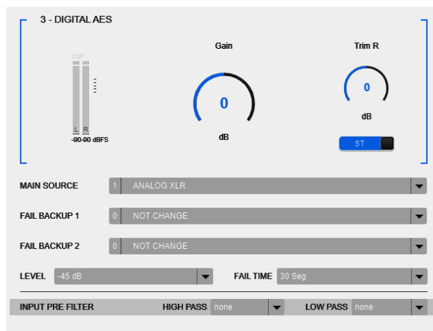
Figura 18: Entrada AES y opciones de conmutación
