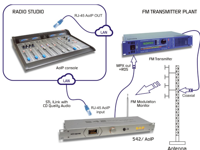
Figura 45: Diagrama básico de conexión por streaming
