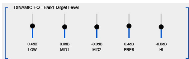
Ilustración 38: MB AGC - Niveles de referencia
