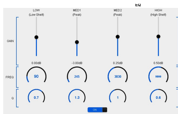
Figura 35: Ecualizador paramétrico de 4 bandas
