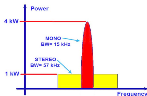
Ilustración 25: Concentración de energía en transmisión mono vs estéreo
