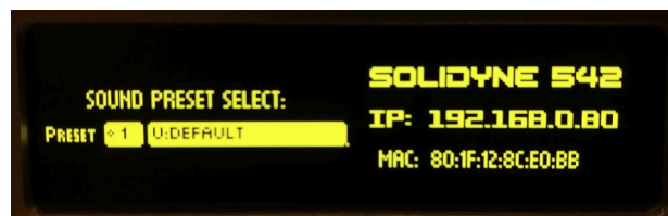
Figura 3: Pantalla inicial
